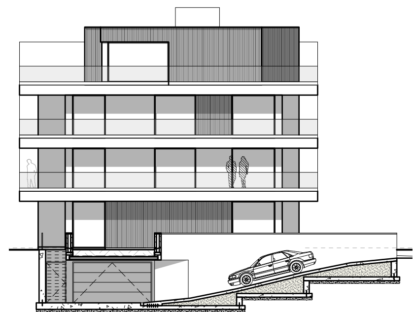
ZIJGEVEL LINKS
